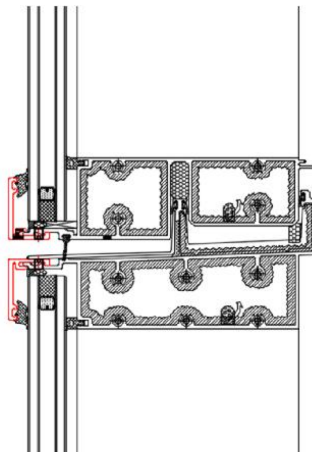
明框形式（无结构胶）
