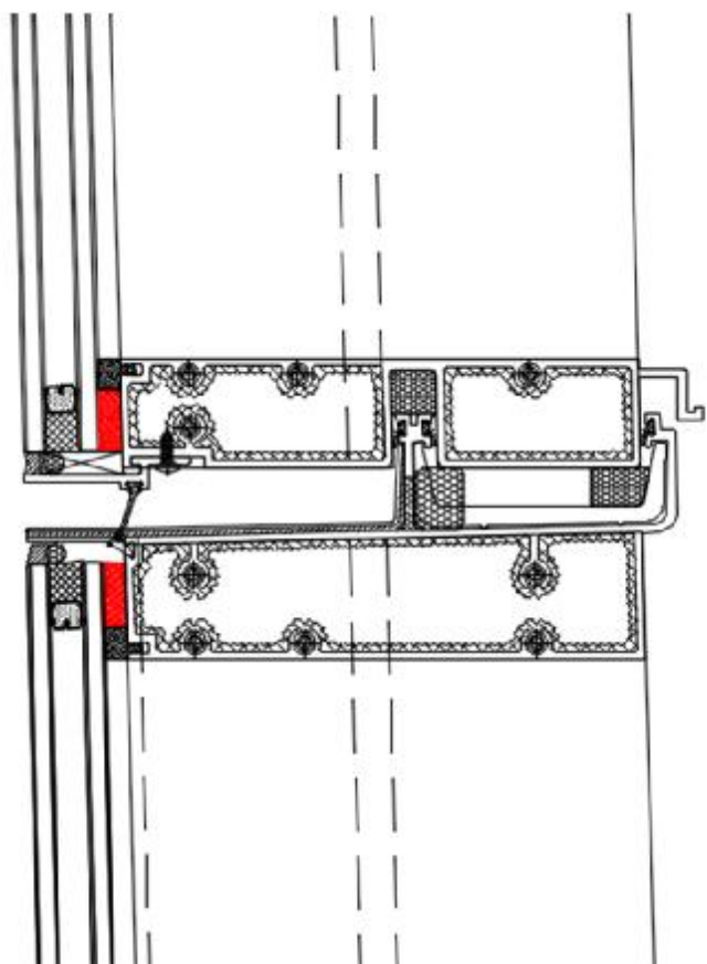
隐框单元体（有结构胶）
